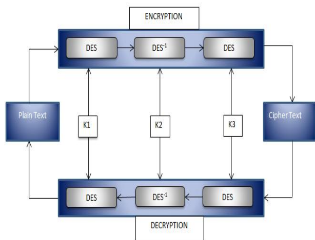
Fig 5: Triple DES
